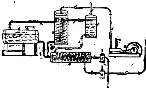
Фиг. 6. Способъ Линде для экономическаго полученія прозрачнаго льда изъ перегнанной воды.
